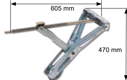
RINFORZATO 1000 KG CORTO SHORT REINFORCED 1000 KG
