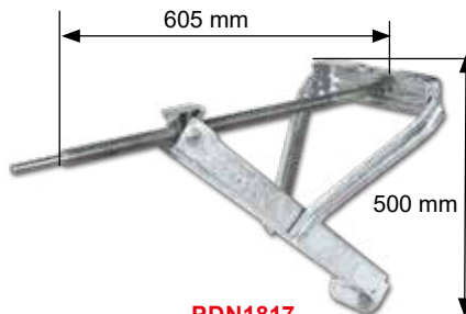
STANDARD 800 KG LUNGO LONG STANDARD 800 KG
