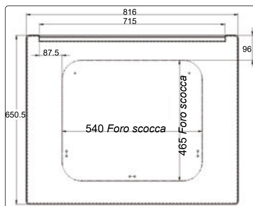
Disegno tecnico FNT6051 Technical drawing FNT6051
